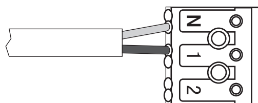
Leuchte - mit Sensor luminaire- with Sensor
