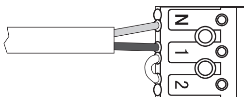
Leuchte - ohne Sensor luminaire- without Sensor
